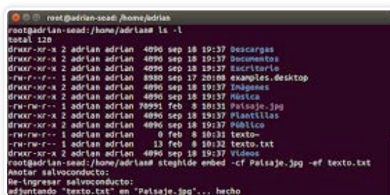
Figura 1: Ocultando fichero de texto en una imagen .jpg con Steghide.
